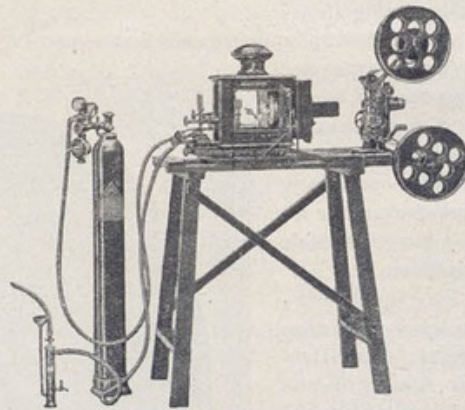
Máquina «Diorama» oxí-aéreo-acetilénica
